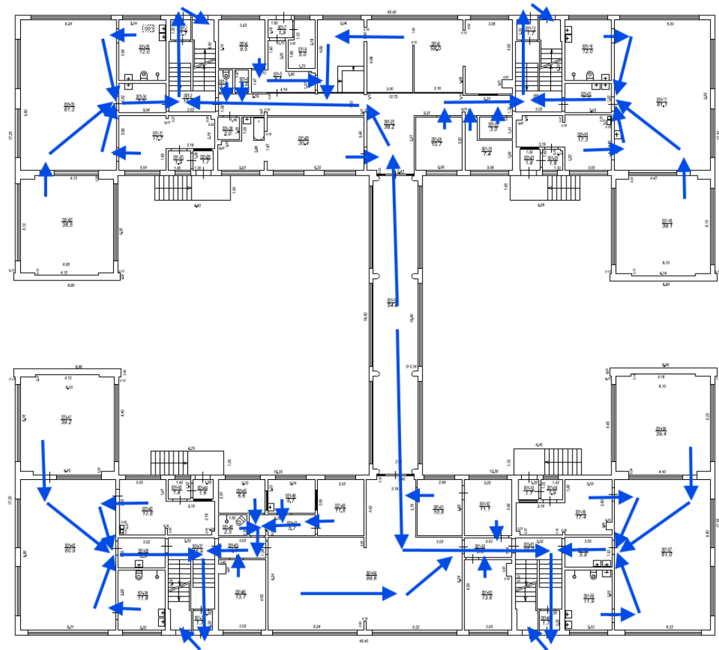
1.stāva plāns
